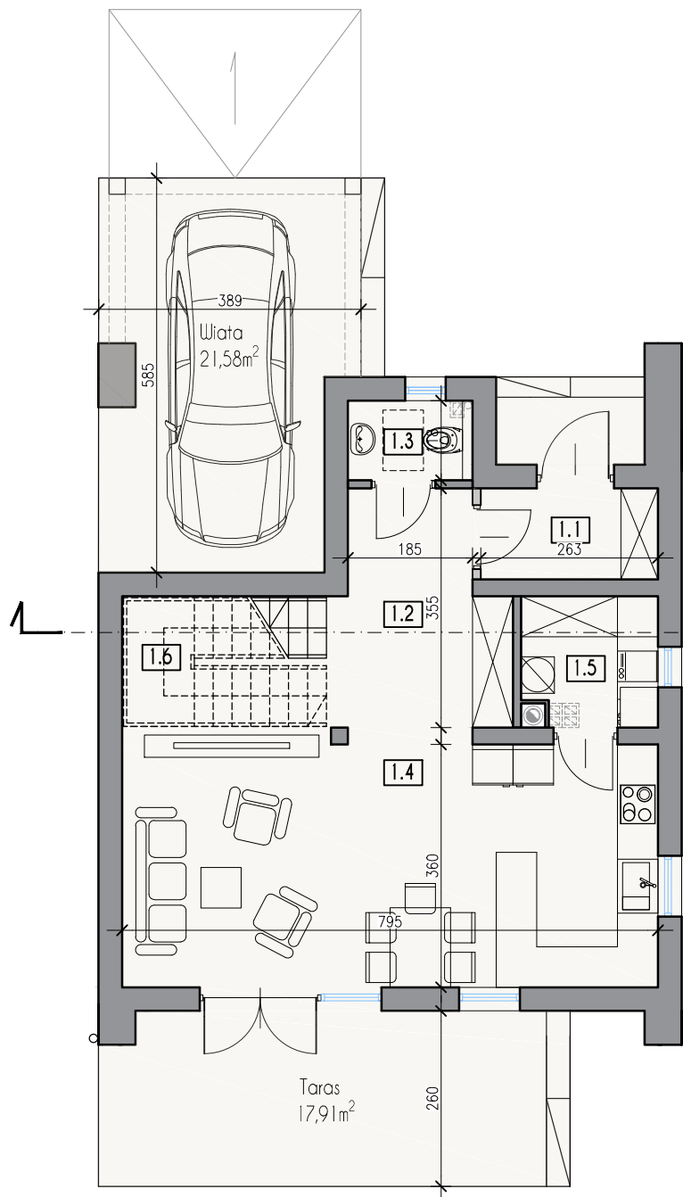
RZUT PARTERU
